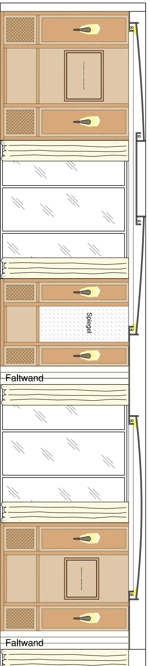
Wandansicht A
